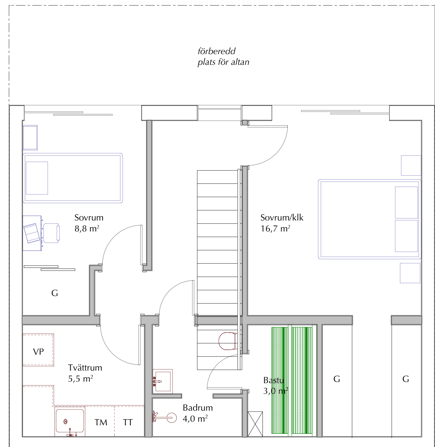
PLAN 1 (alternativ planlösning)
